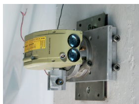
Distancemètre sur support goniométrique (CEREMA)
