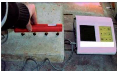
Dispositif Wenner (CEREMA)
